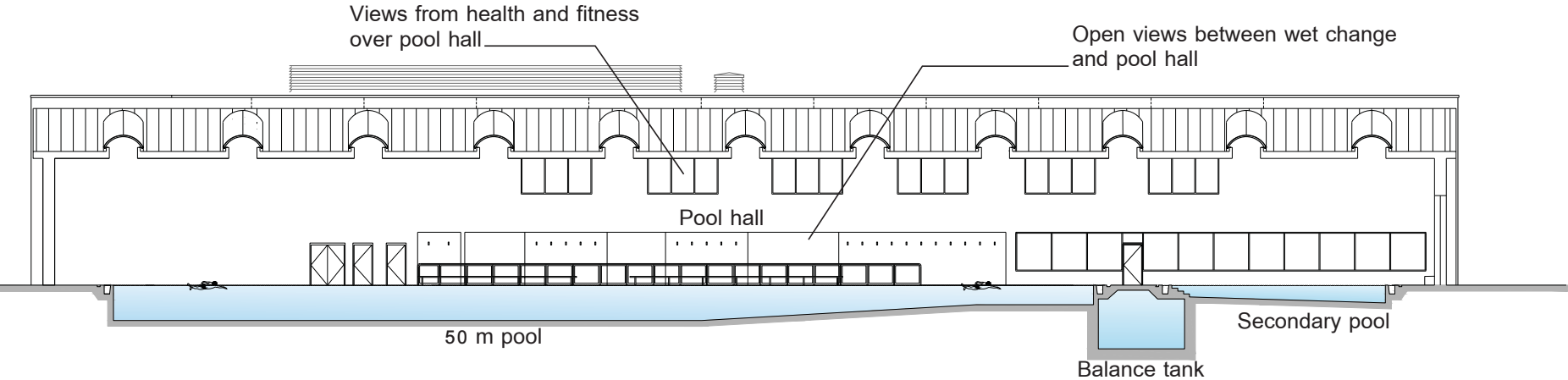
Longitudinal Section
